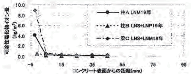
図5 曝露19年後の可溶性塩化物イオン量
