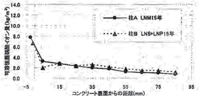
図6 曝露15年後の可溶性亜硝酸イオン量
